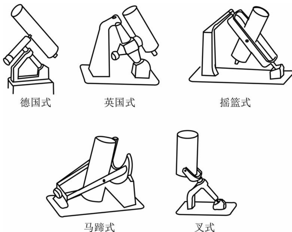
图11 望远镜的装置图
