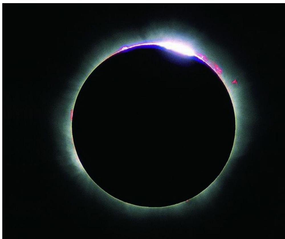
图29 摄影师Luc Viatour在1999年法国日全食时拍到的贝丽珠 ( www.Lucnix.be )
