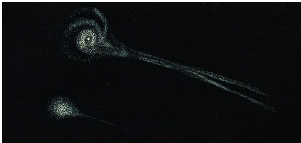
图59 比拉彗星
