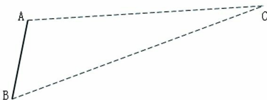
图56 用三角测量法测不能准确测出遥远物体的距离
