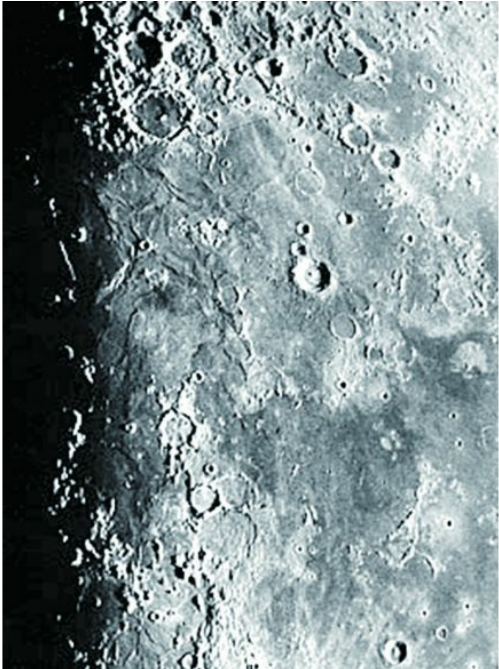
图22 月亮的表面
