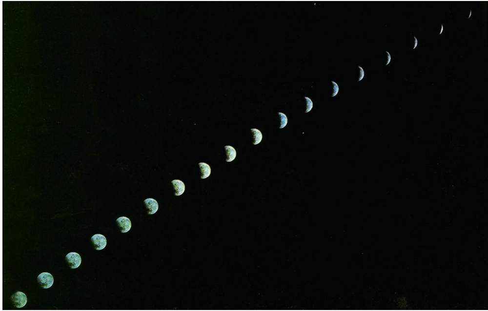
图26 月食全过程
