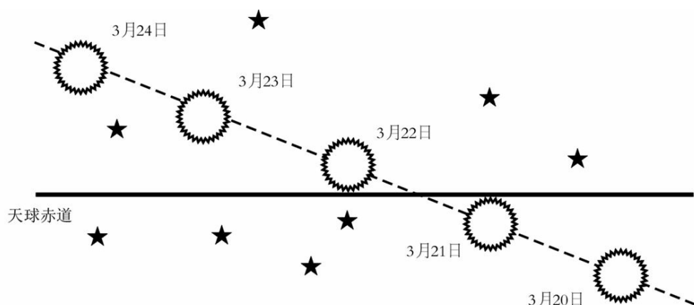
图4 太阳于3月21日前后经过赤道
