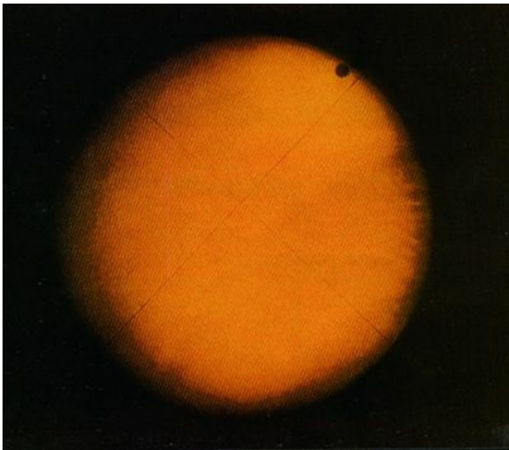
图36 金星凌日
