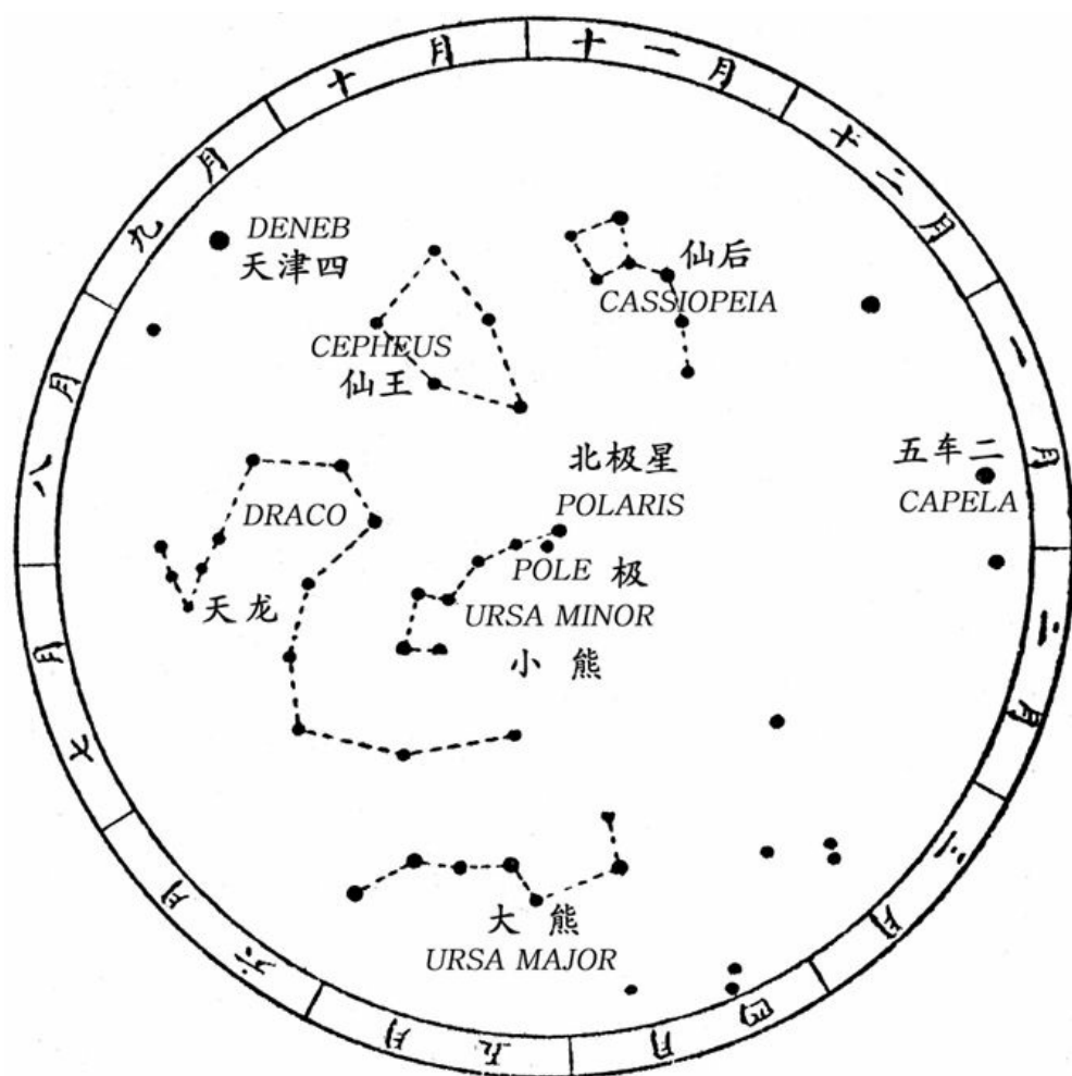
图2 北天与北极星
