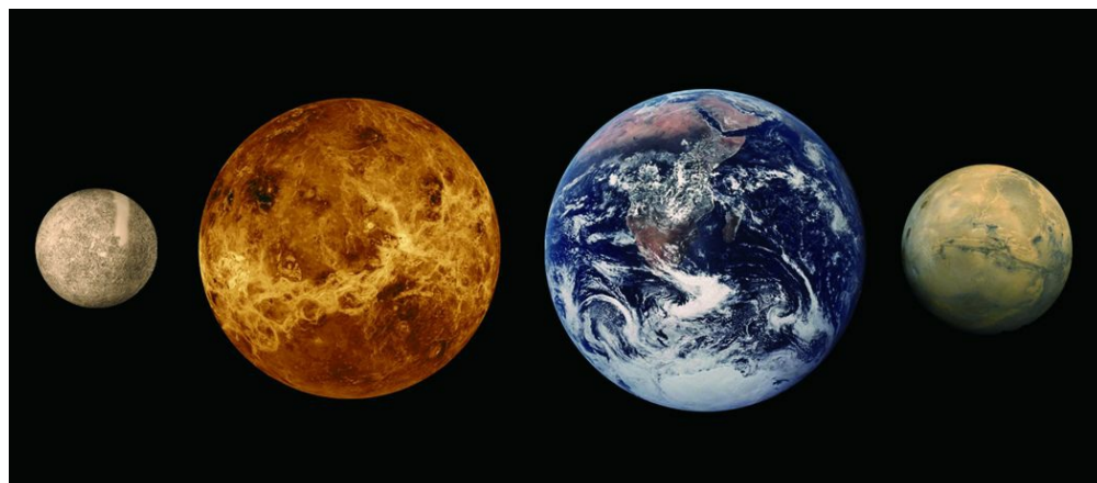
图15 类地行星（从左至右依次为：水星、金星、地球、火星）
