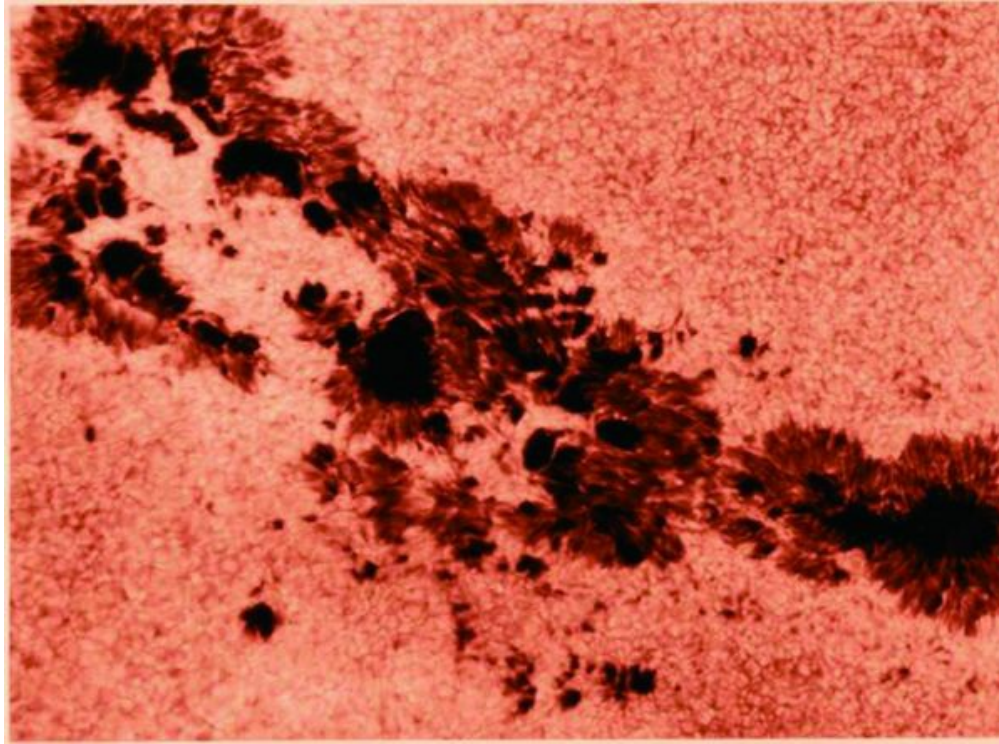
图16 带黑子的太阳光球（上）及太阳黑子详图（下）
