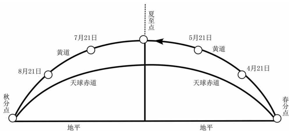
图8 3月到9月间太阳的视运动
