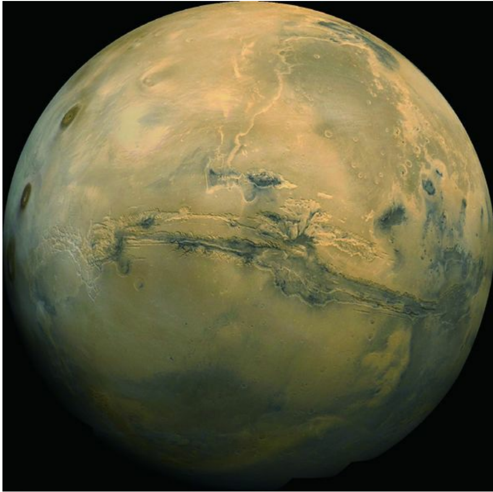
图38 火星的『运河』
