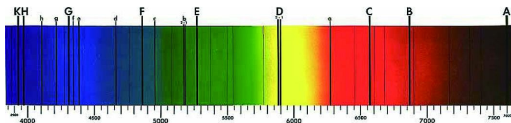
图70 夫琅和费谱线
