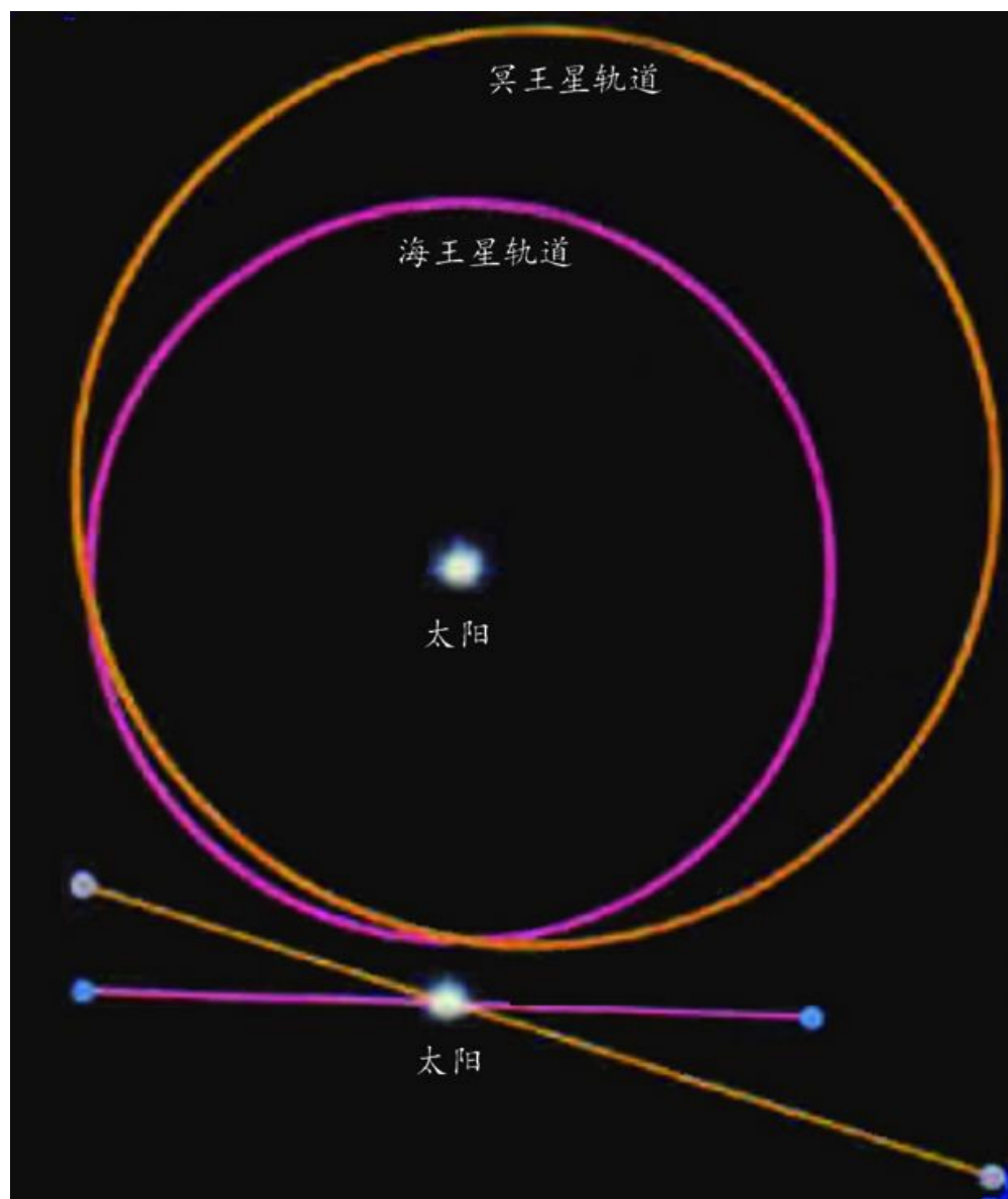
图55 冥王星的轨迹
