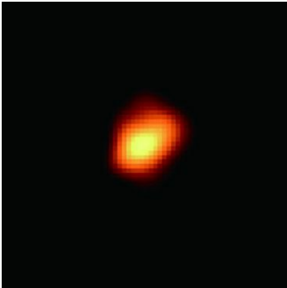
图73 （左）蒭藁增二
