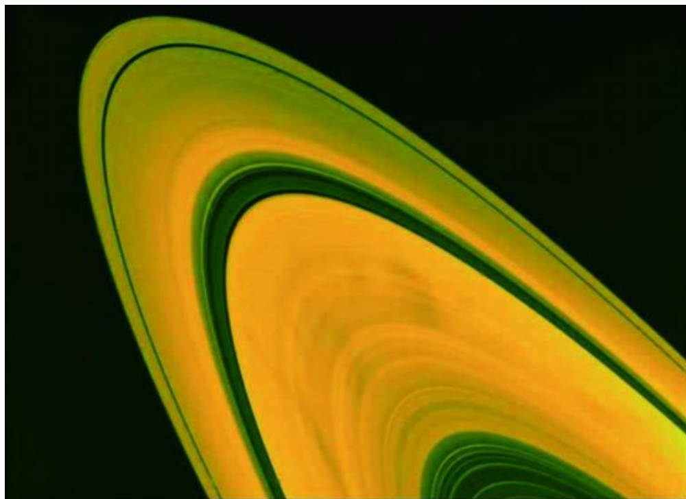
图47 土星光环详图
