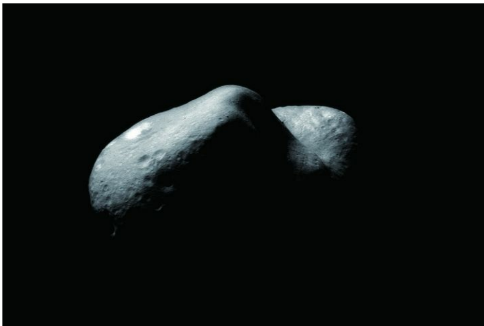
图43 爱神星
