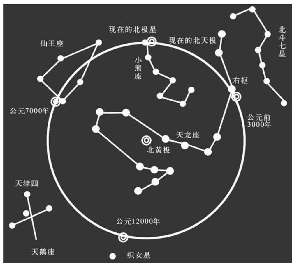
图9 岁差
