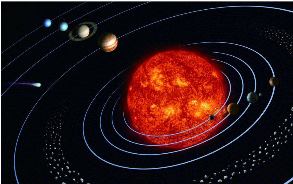
图14 太阳系
