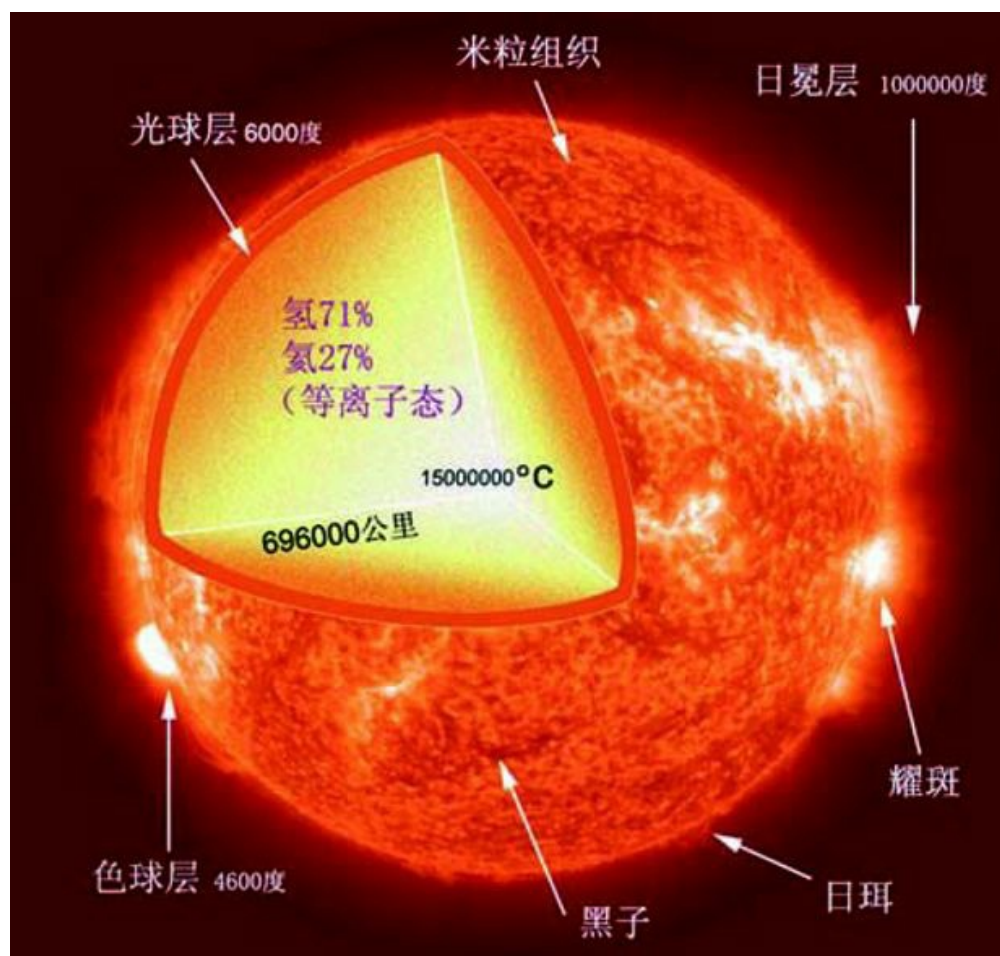
图18 太阳的结构
