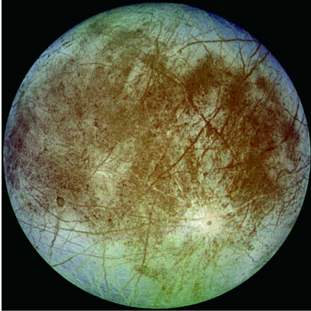
图46 木卫二
