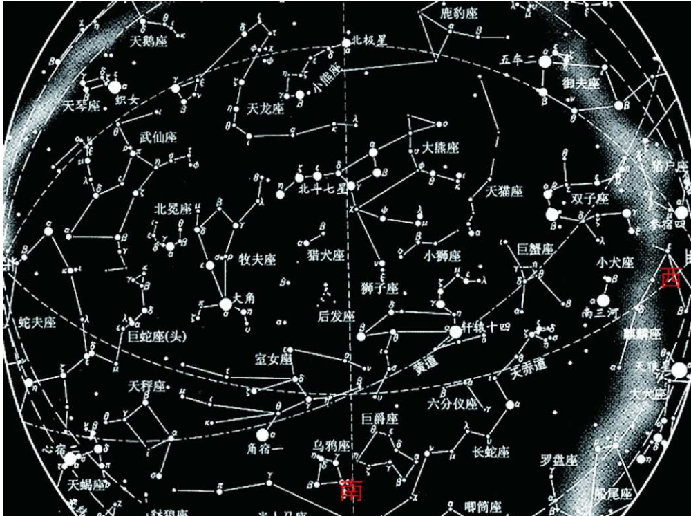
图68 春季星座
