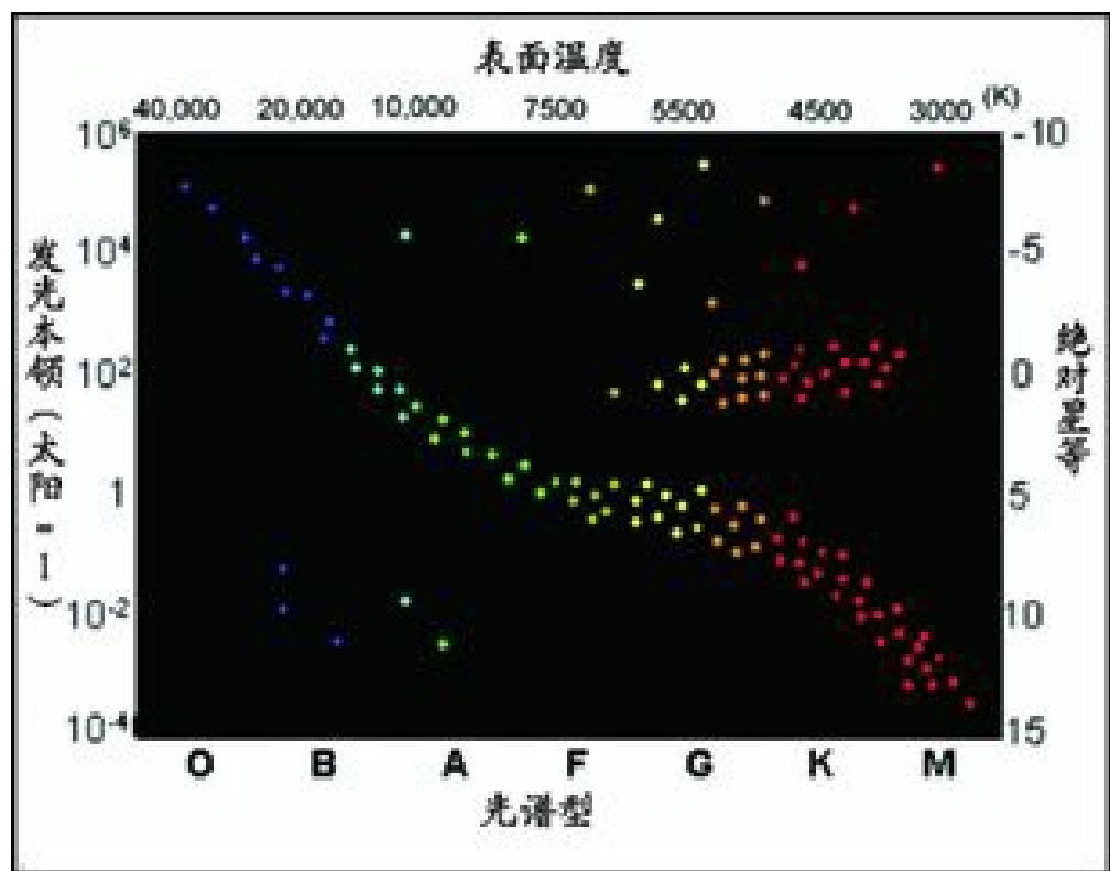
图71 光谱——发光本领图解
