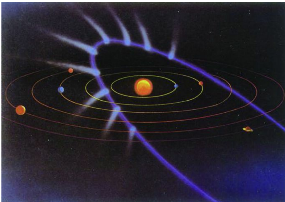
图57 彗星的抛物线轨道
