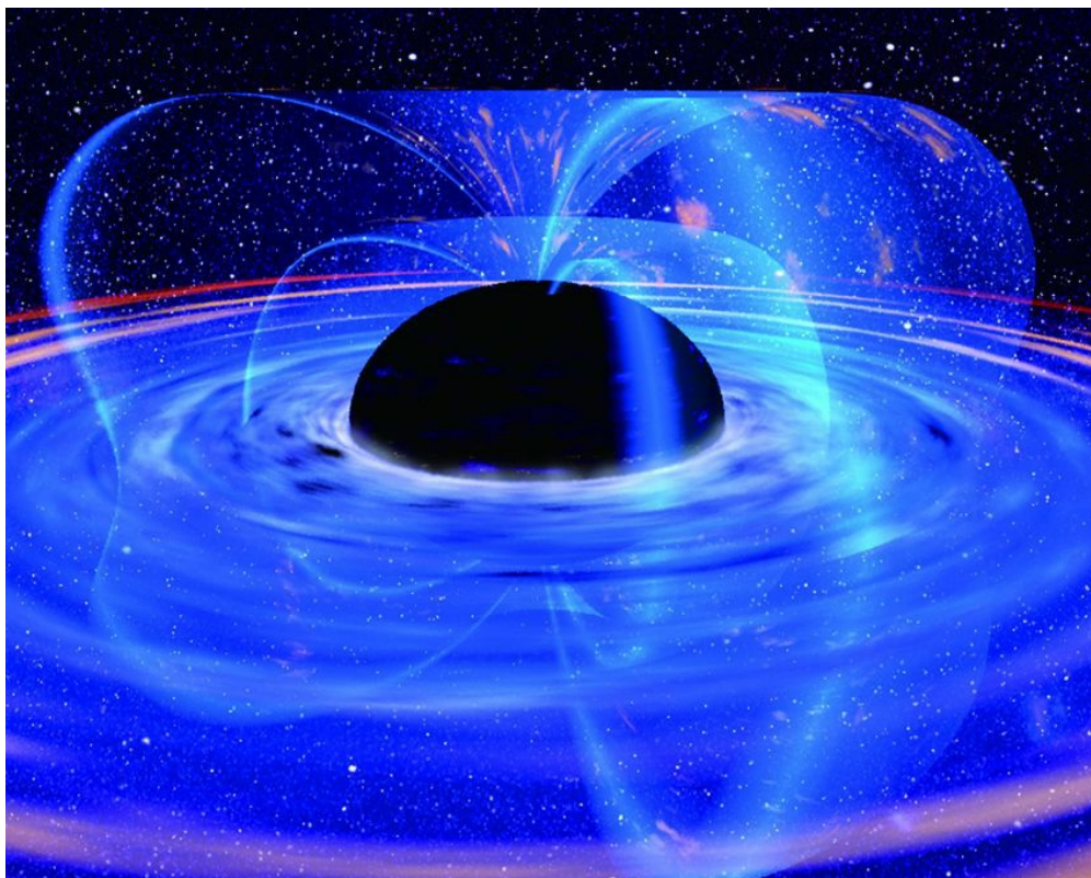
图78 黑洞模拟图
