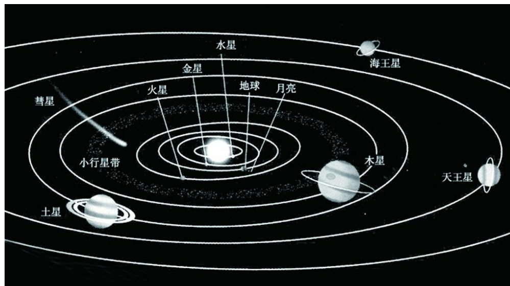
图30 太阳系天体
