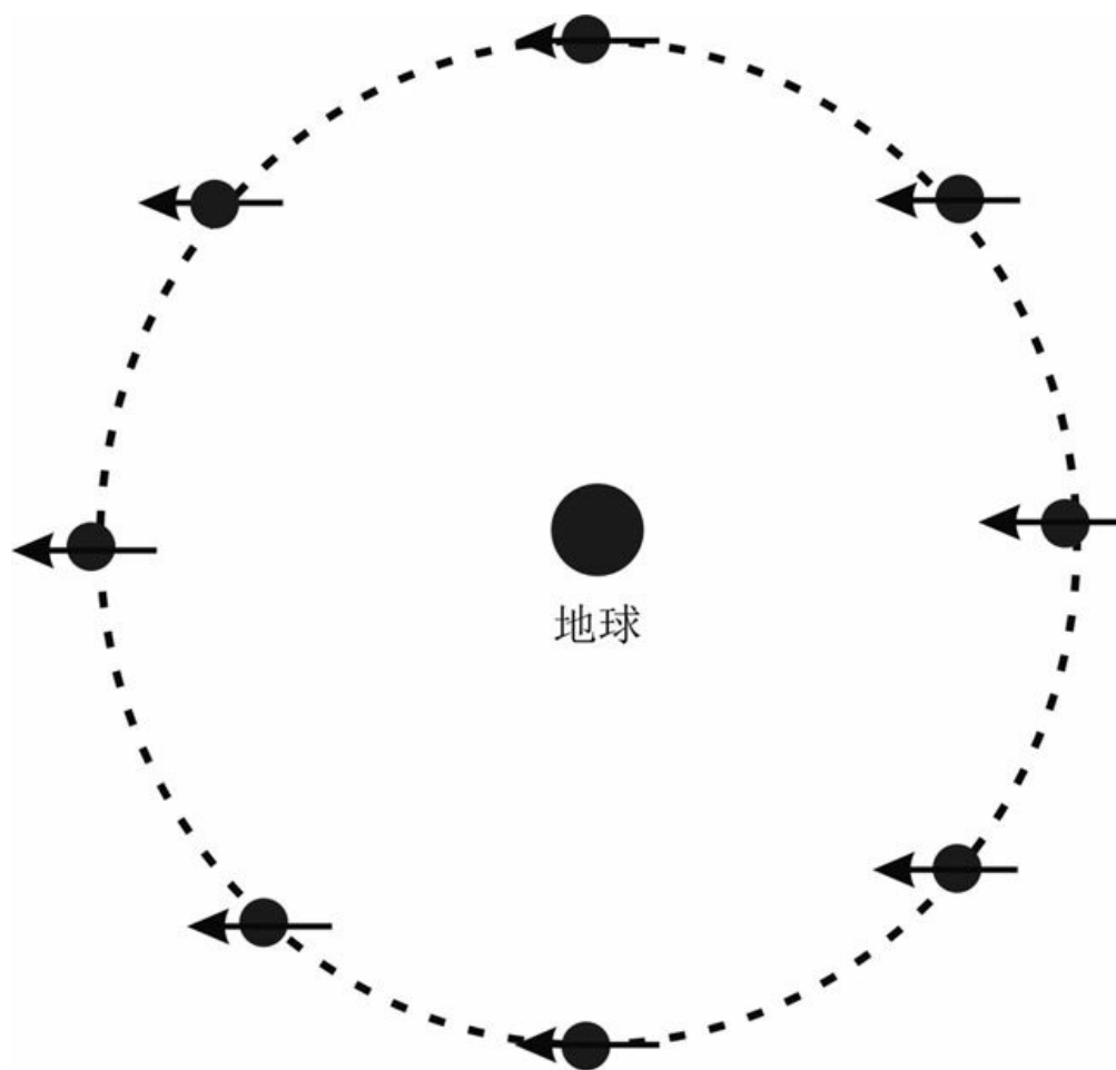
图23 假如月亮不自转时月亮的运动
