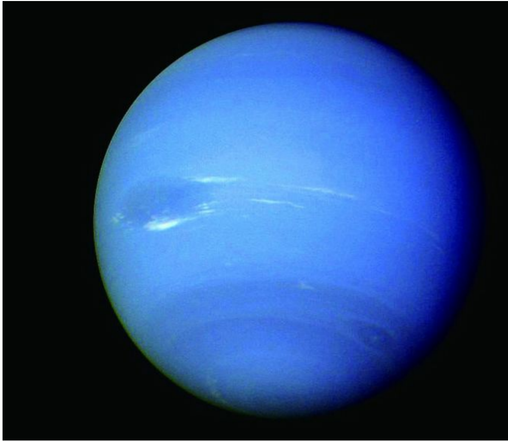
图53 旅行者2号航天器拍到的海王星
