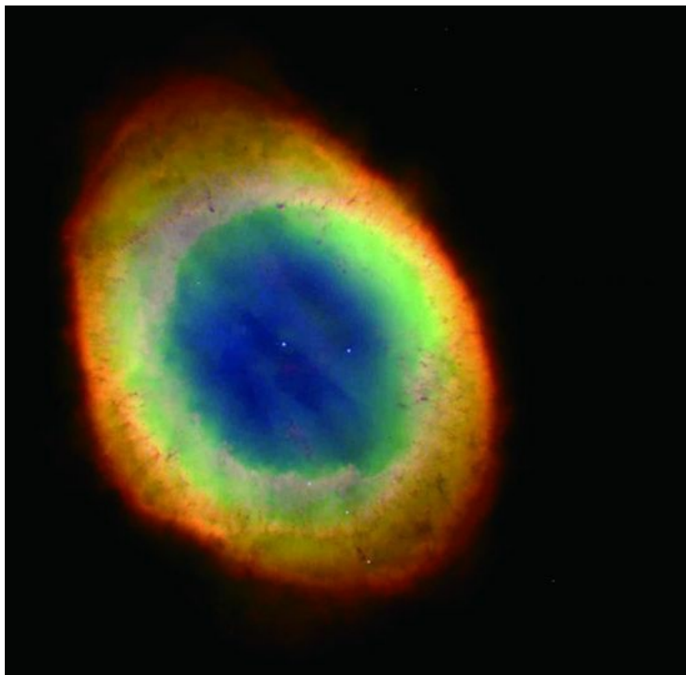
图89 天琴座环状星云
