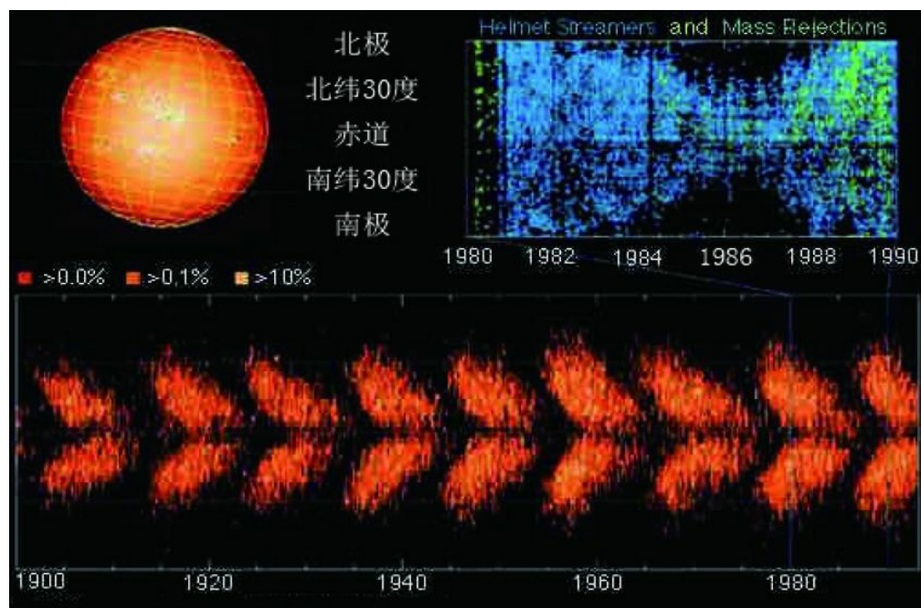
图17 太阳黑子的纬度分布
