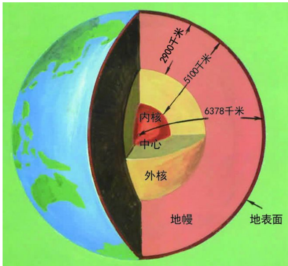
图20 地球的结构
