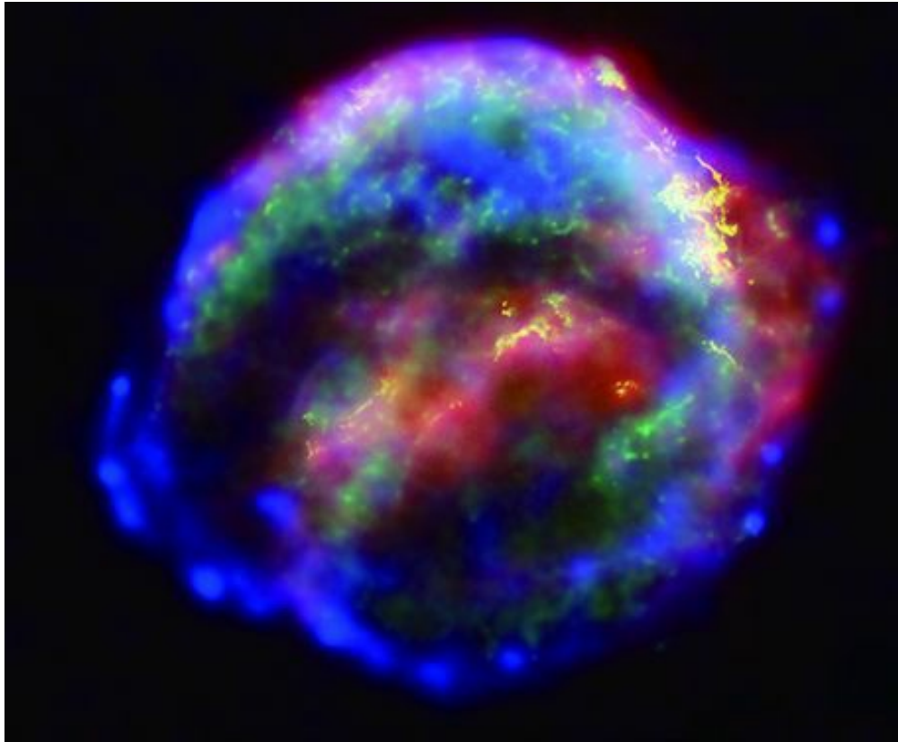
图76 （右）开普勒超新星爆发后的遗骸
