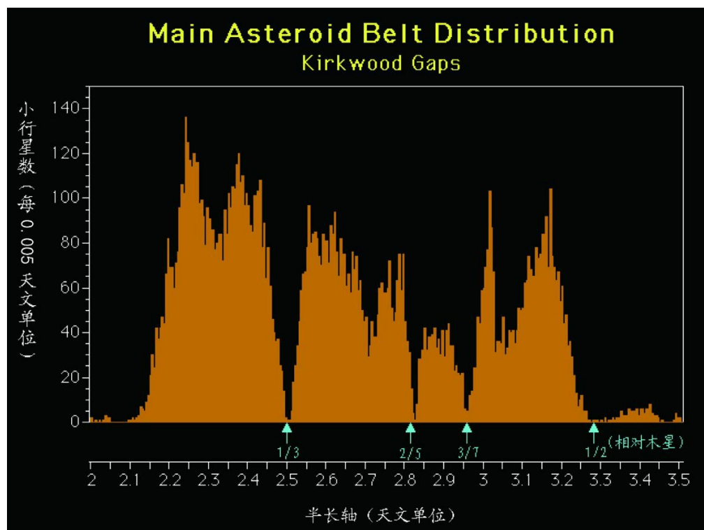
图42 小行星轨道的分布
