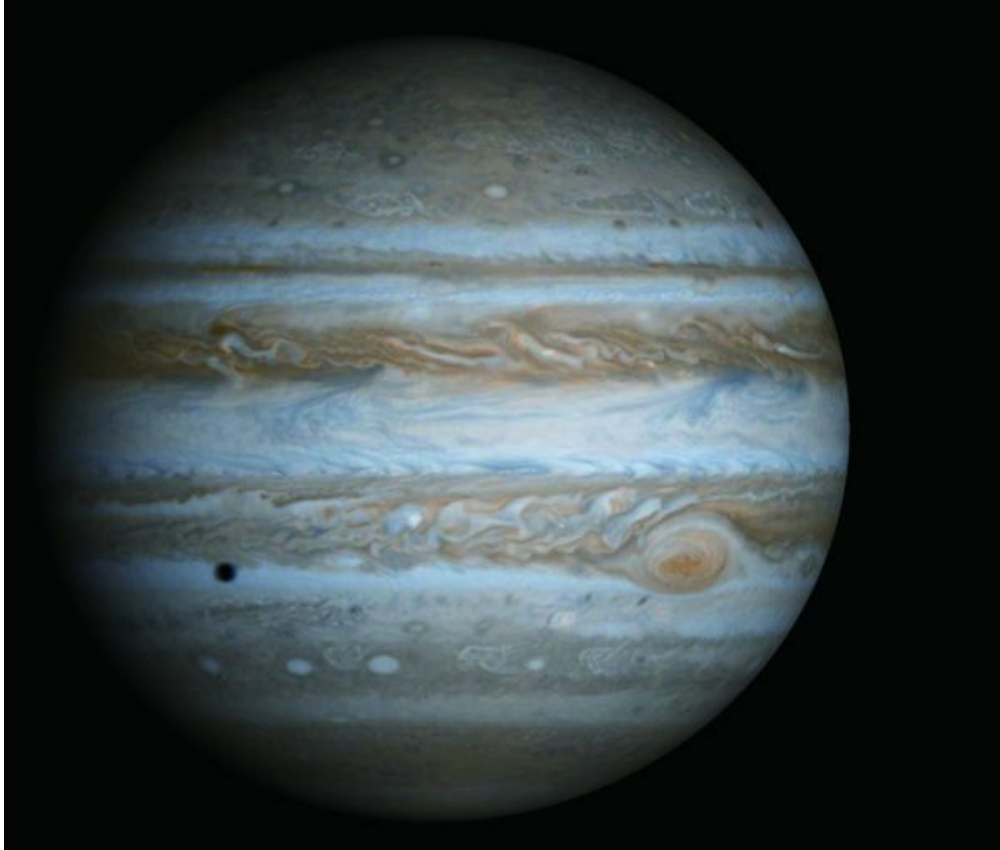
图44 木星
