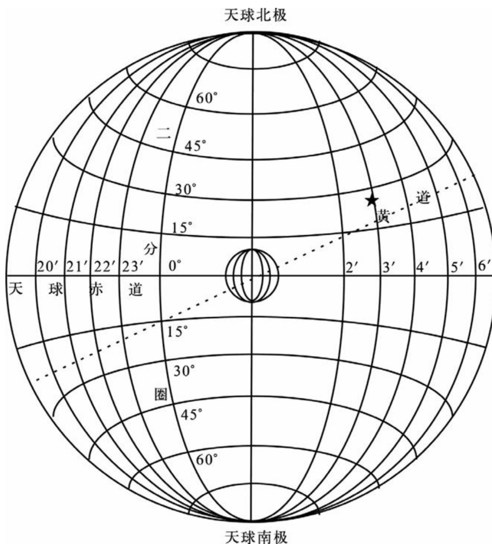
图3 天球的经纬
