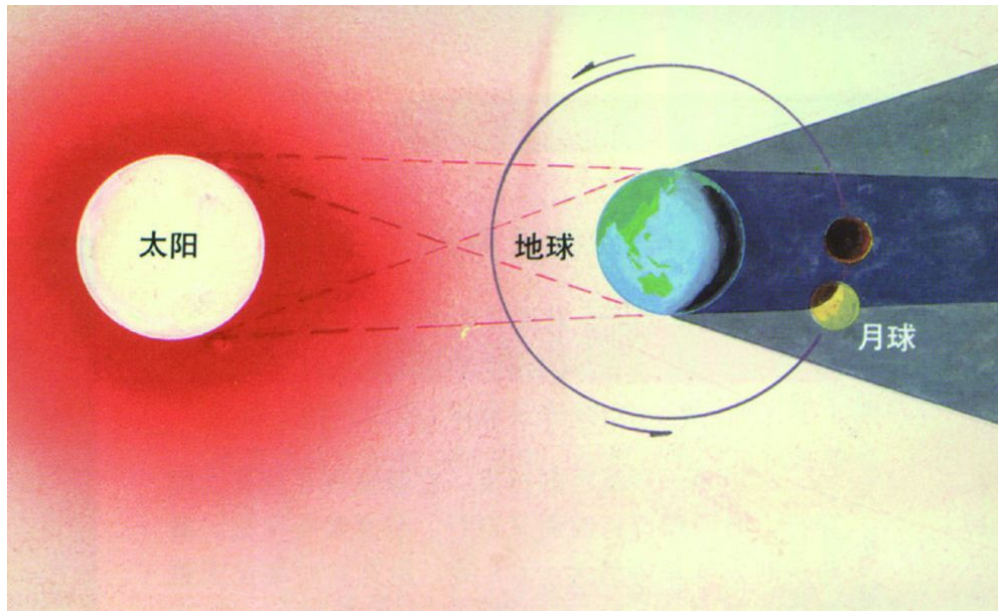
图25 月亮在地球暗影中
