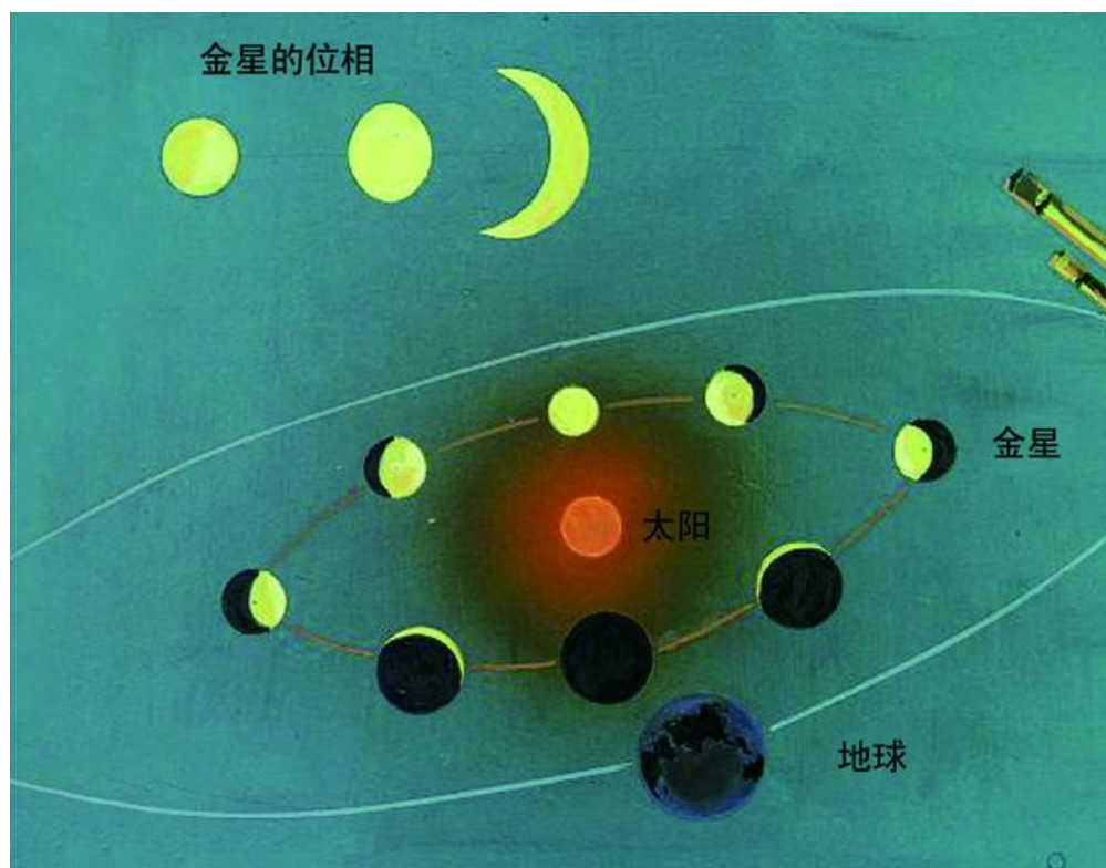
图34 金星在轨道中各点的位相
