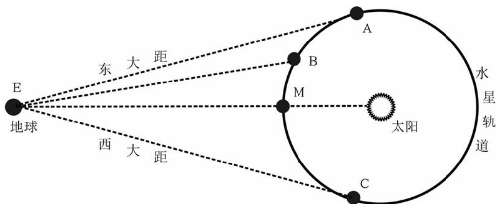
图32 水星的距角
