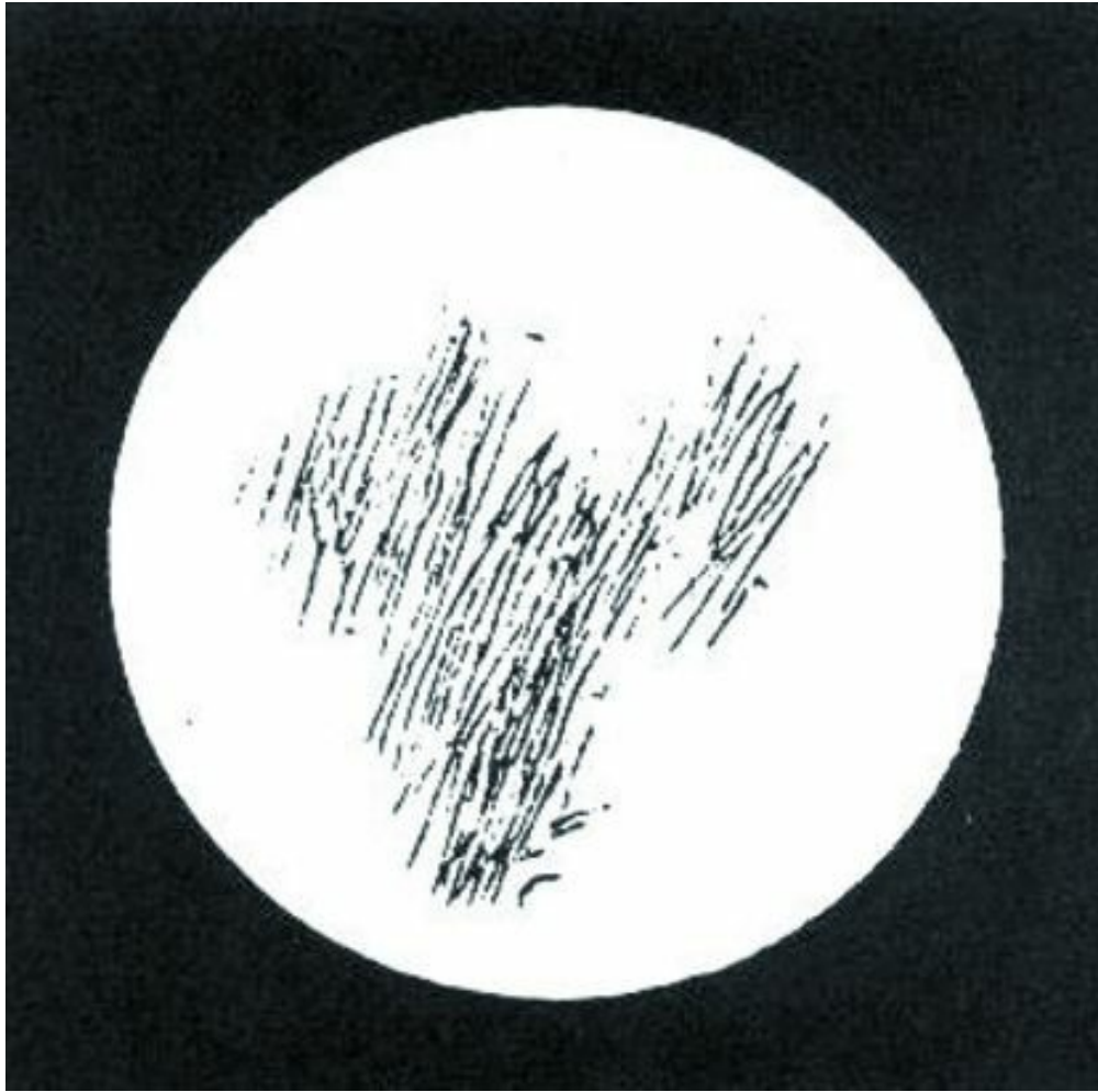
图37 惠更斯笔下的火星
