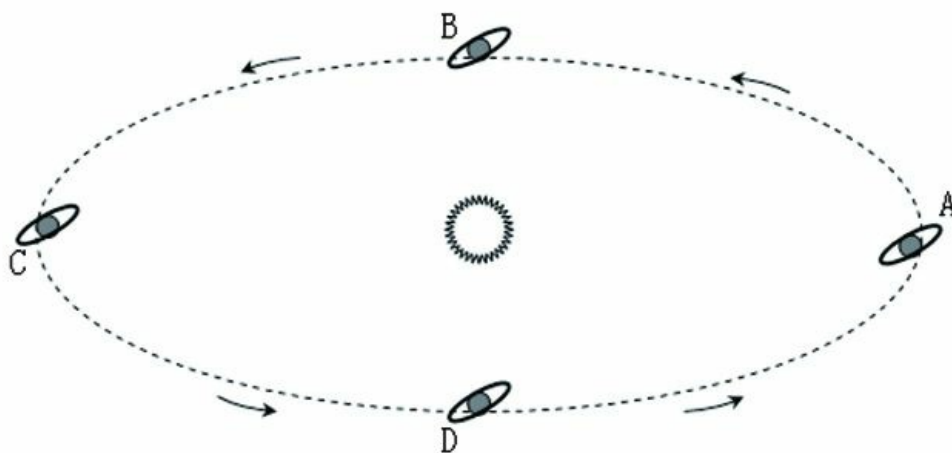
图49 倾斜的土星光环
