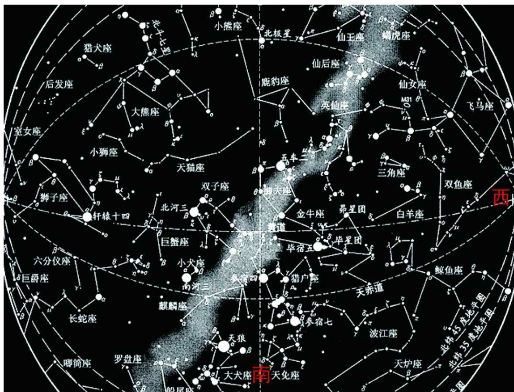
图67 冬季星座
