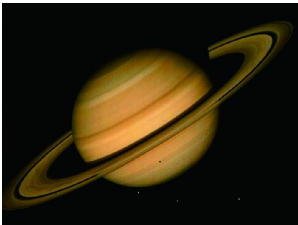
图47 土星光环详图
