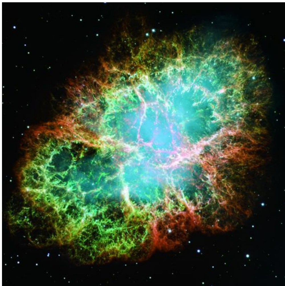
图77 蟹状星云脉冲星所在的蟹状星云
