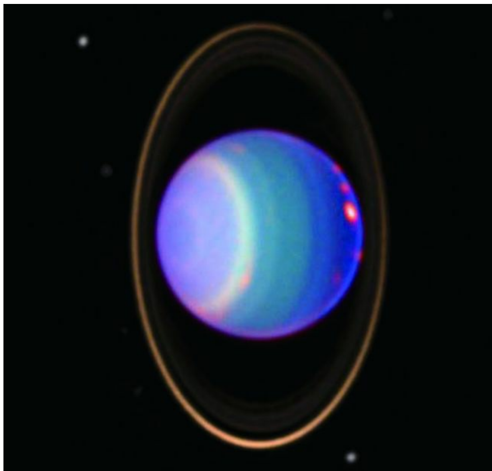
图52 哈勃太空望远镜拍到的天王星影像
