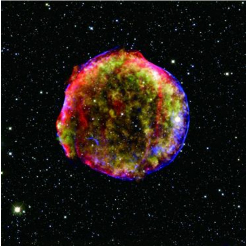
图75 （左）第谷超新星
