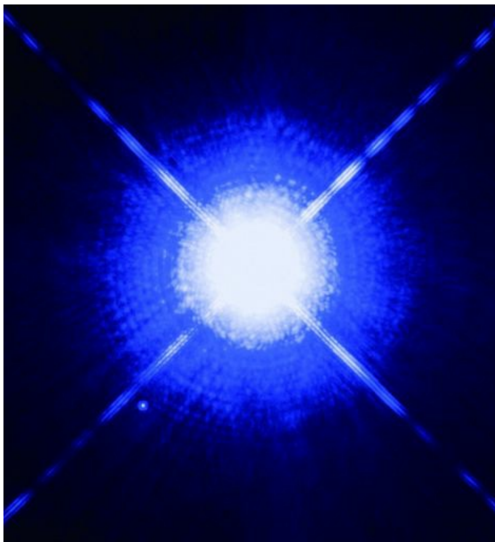
图72 哈勃太空望远镜拍摄的天狼星A和天狼星B（左下方的伴星天狼B为白矮星）
