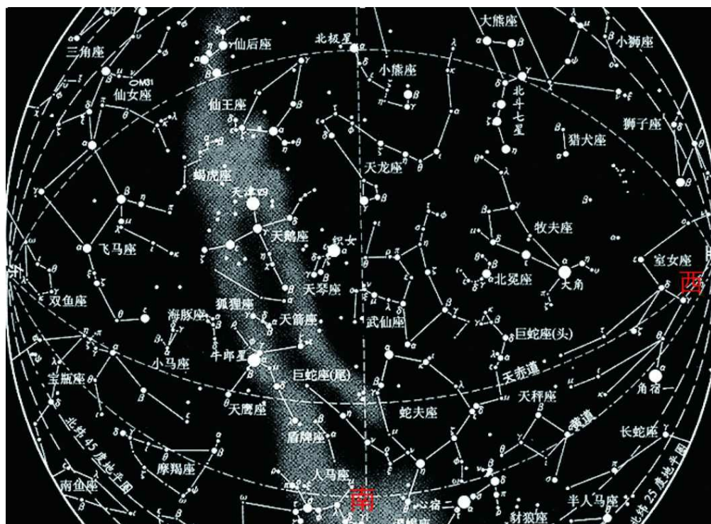
图69 夏季星座
