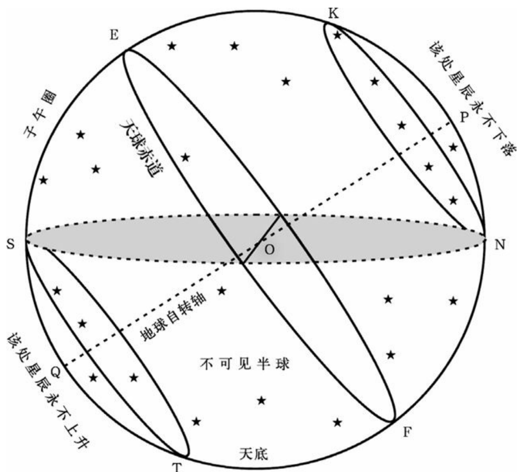
图1 我们眼中的天球
