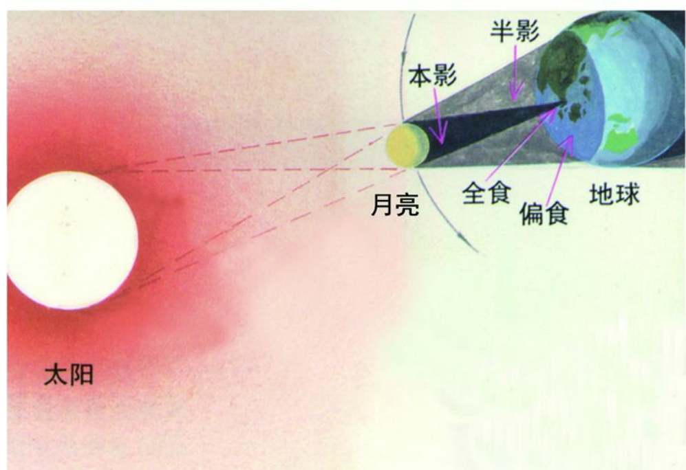
图27 日食形成示意图
