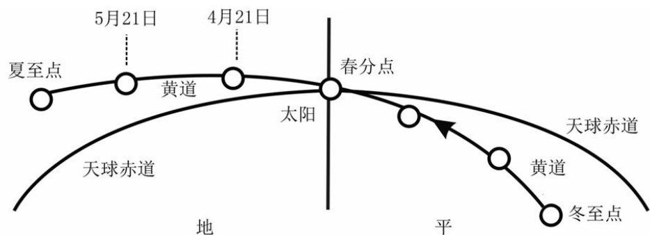
图7 春夏间太阳沿黄道的视运动
