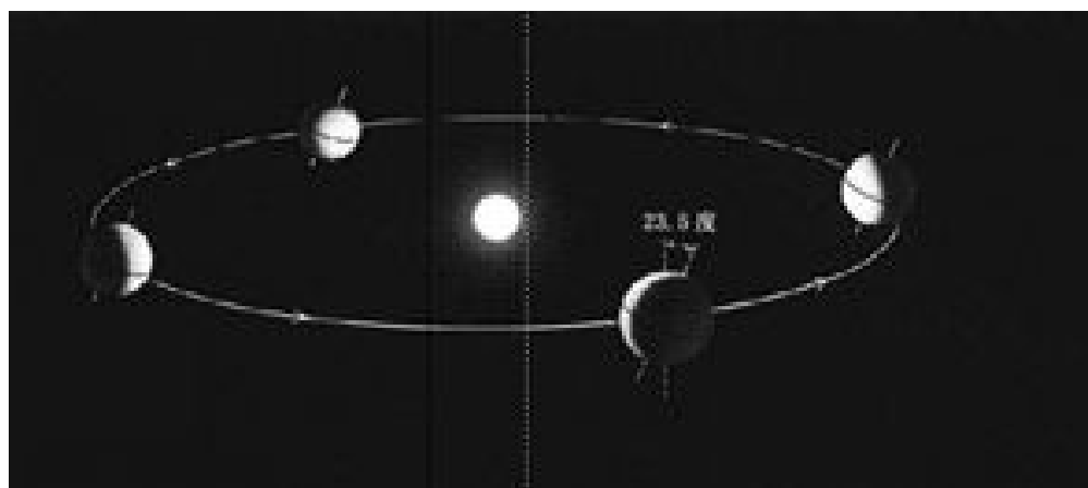
图6 如何因黄道倾斜而有四季
