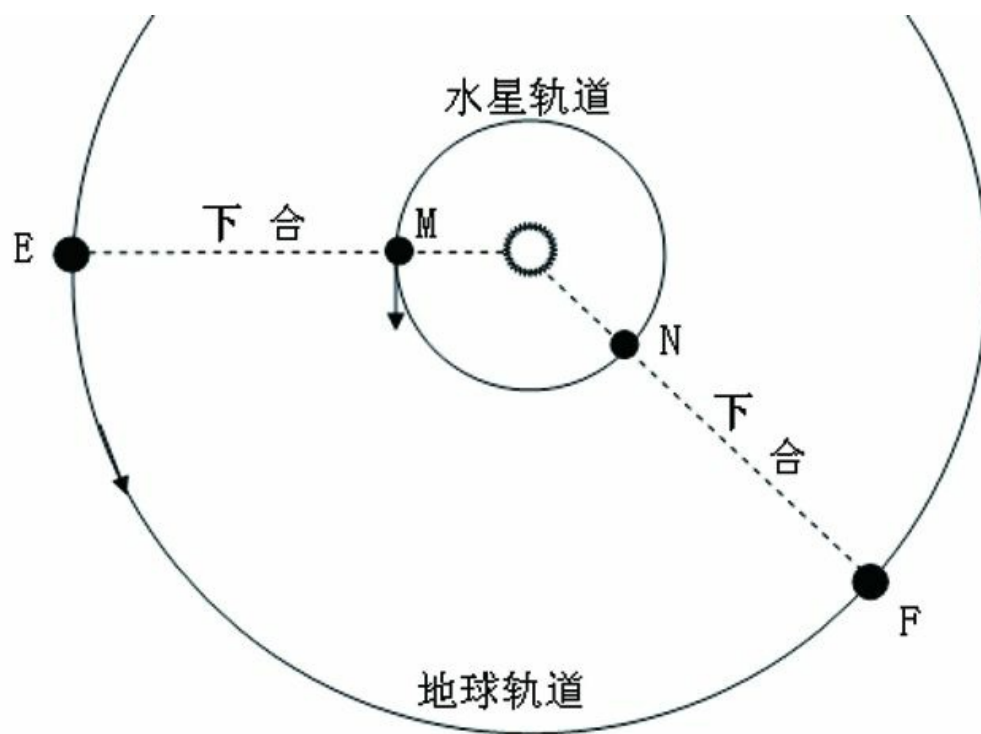
图31 水星合日
