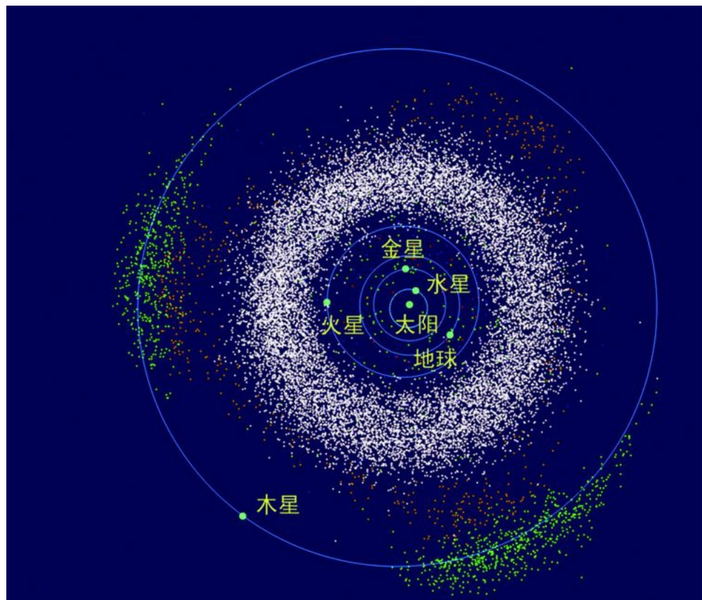
图41 主小行星带（白色部分）
