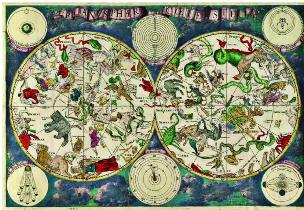
图64 弗雷德里克·德·威特于1670年绘制的星座图
