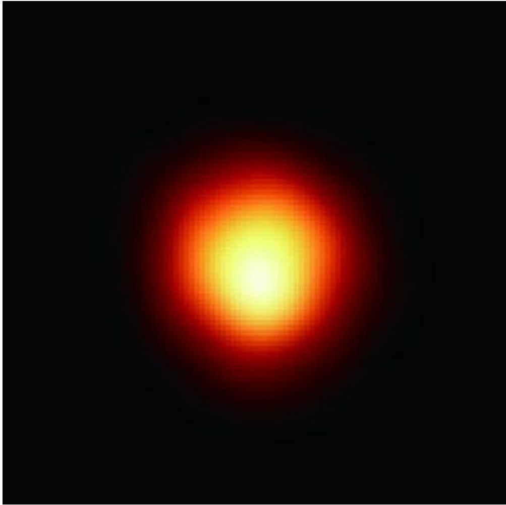
图74 （右）参宿四
